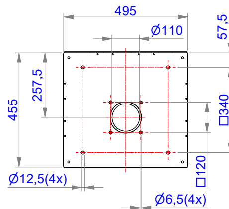
A-A ( 1 : 15 )
