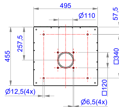
A-A ( 1 : 15 )
