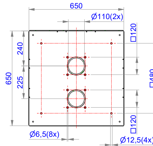
A-A ( 1 : 15 )
