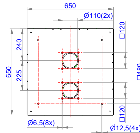
A-A ( 1 : 15 )
