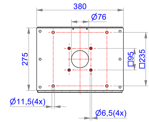
A-A ( 1:10 )
