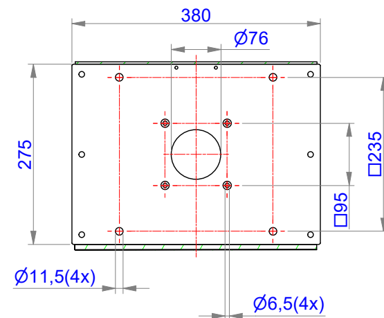
A-A ( 1:8 )
